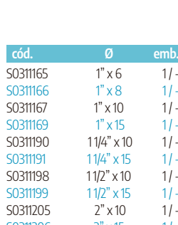
Tapa polipropileno M
