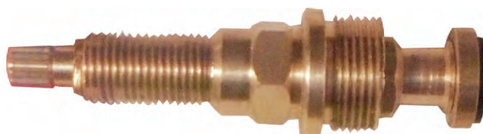
Cabezal Fv artesanal lateral bañera
