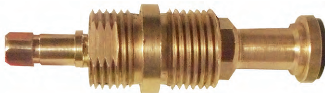
Cabezal Peirano no ascendente
