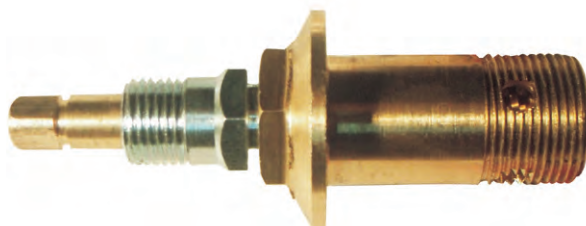
Cabezal Peirano transferencia lluvia grande
